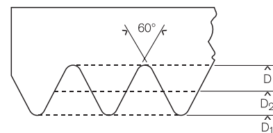
D 1 Prečnik jezgra D 2 Prečnik bokova D Nazivna mera navoja/ spoljnog prečnika
