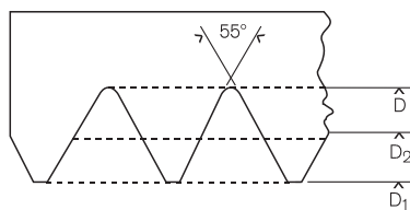
D 1 Prečnik jezgra D 2 Prečnik bokova D Nazivna mera navoja/ spoljnog prečnika
