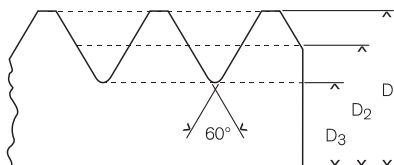
D 3 Prečnik jezgra D 2 Prečnik bokova D Spoljni prečnik
